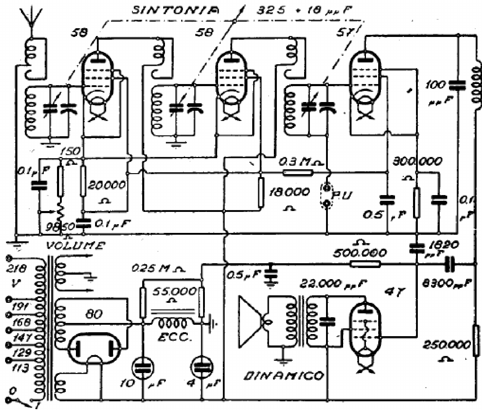
COMPAGNIA GENERALE DI ELETTRICITA' - MOD. « RADIETTA 53 »
